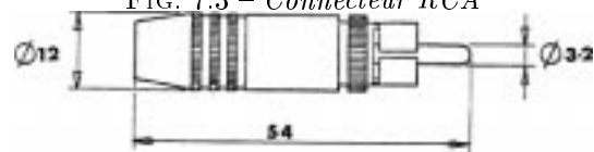
FIG. 7.4 – Connecteur RCA
