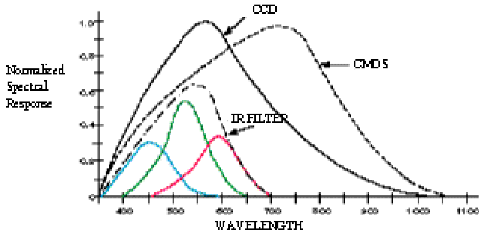
FIG. 3.10 – Spectre du capteur en fonction de filtres couleur
