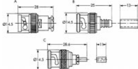
FIG. 7.1 – Connecteur BNC
