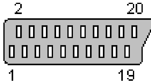
FIG. 7.7 – Prise PÉRITEL
