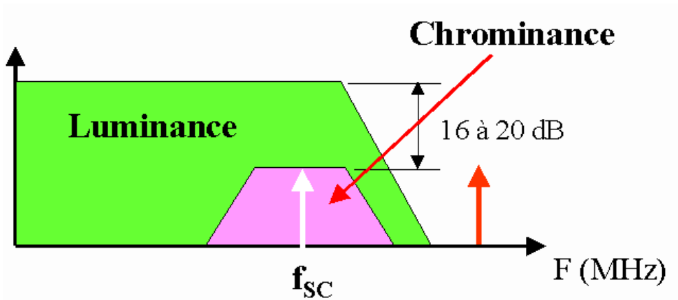
FIG. 4.2 – Modulation de la chrominance et de la luminance
