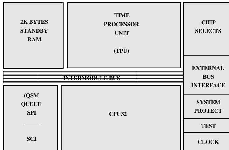
FIG. 2.3: Sch ma block du MC68332
