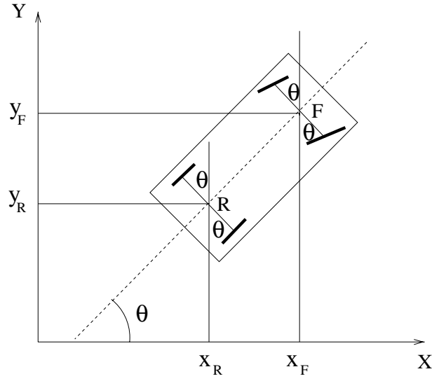
FIG. 4.3: Mise en  vidence de l'orientation \theta aux centres des essieux.
