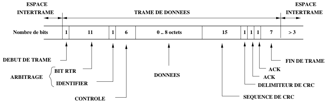
FIG. 2.8: Protocole CAN: la trame de donn es
