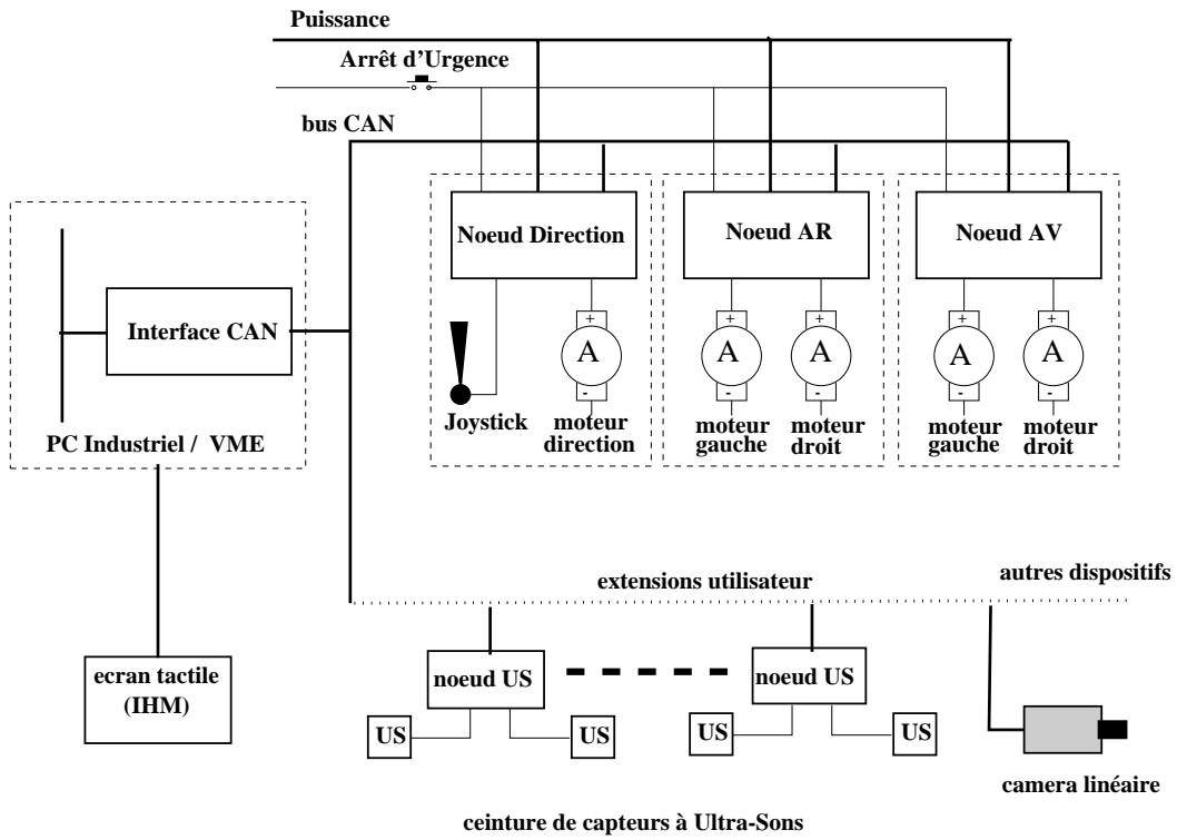
FIG. 1.2: Synoptique de l'architecture matérielle de Contrôle/Commande
